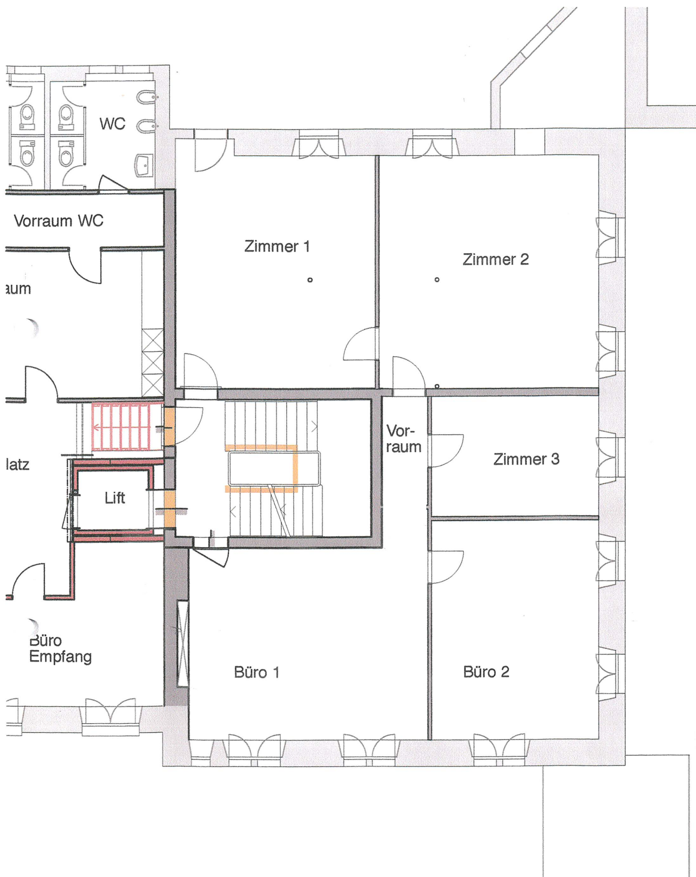
2. OBERGESCHOSS
